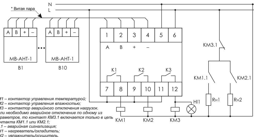
Схема подключения с контакторами
